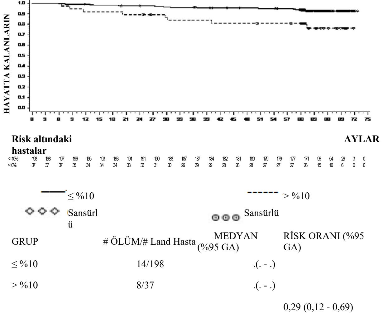
Şekil 4: Yeni kronik evre KML tanısı almış olan hastalarda yapılan bir faz 3 çalışmada 3. ayda BCR-ABL düzeyine ( \leq \%10 veya > \%10 ) göre dasatinib'in genel sağkalım için sınır noktası grafiği
